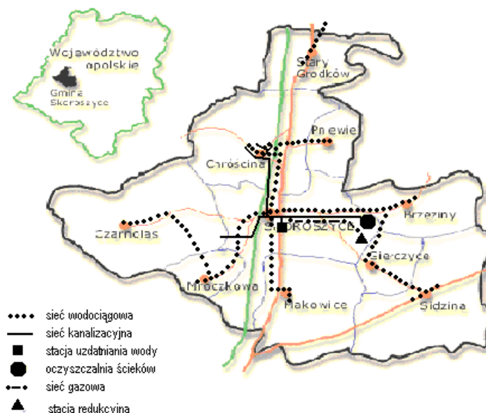
Rys. 2. Infrastruktura techniczna Gminy Skoroszyce
